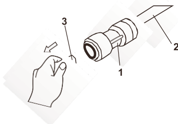
Conector de agua
