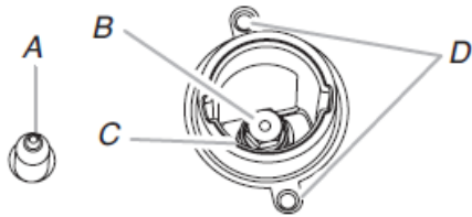
A. Électrode d'allumage B. Injecteur C. Porte-injecteur à orifice D. Vis
