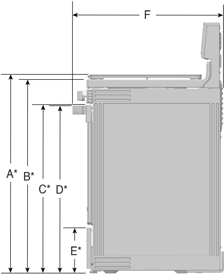
VUE LATÉRALE
