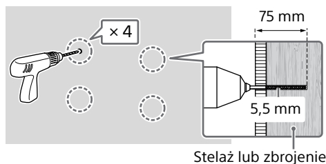
Stelaż lub zbrojenie
