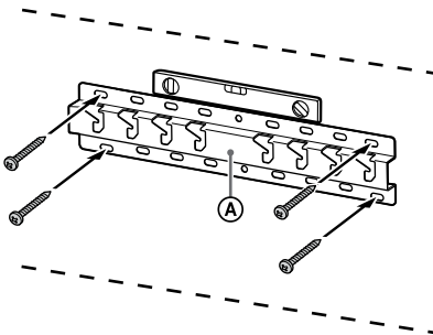
مثال: نصب پایه (20) A در محل "a"
