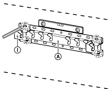
Exemplu: Marcarea poziției „a” pentru a montarea bazei (20) ③
