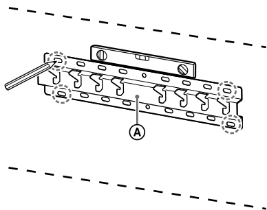
Příklad: označení na místě „a“ pro osazení základny (20) ①
