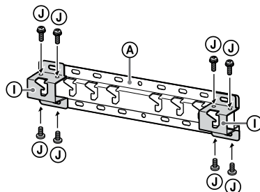
Пример: Монтиране на адаптера на основата ① в позиция "а"
