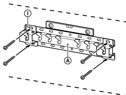
Příklad: osazení základny (20) ① na místě „a“
