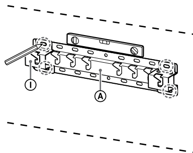
Пример: Маркиране на позиция "а" при монтиране на основата (20) ④
