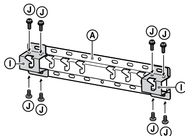
Pvz., pagrindo adapterio ① tvirtinimas „a“ taške
