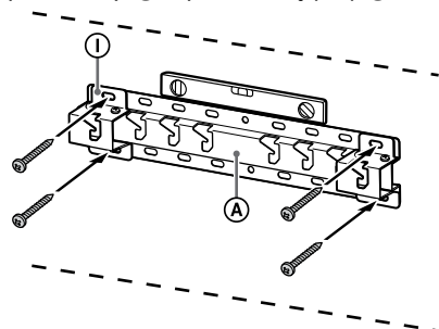
Przykład, montażu podstawy (20) A w miejscu „a”
